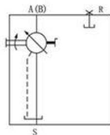
手动变量MA Manual control
