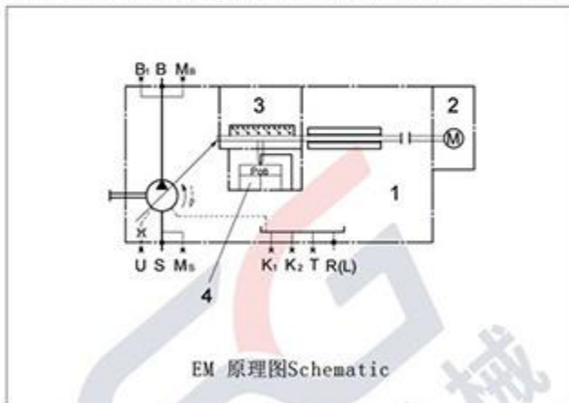
图中元件 Diagram components
