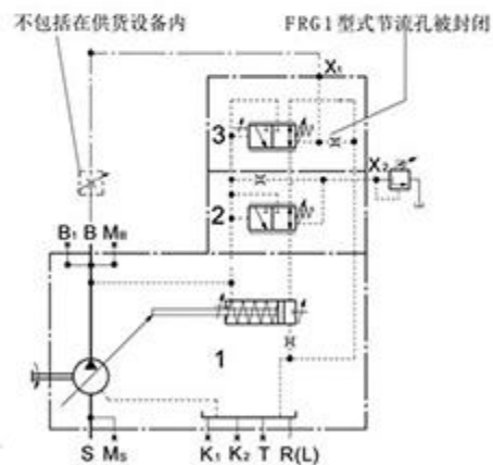
FRG 原理图Schematic
