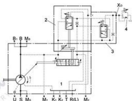
LR2G 原理图Schematic
