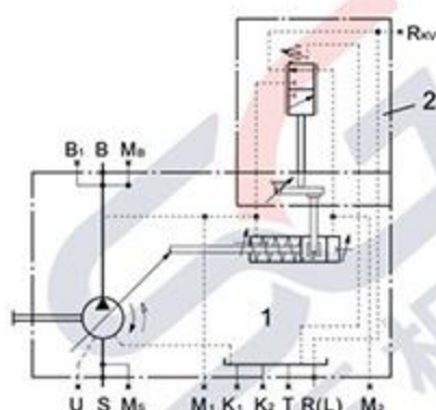
LR2 原理图Schematic
