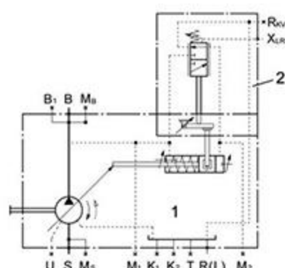
LR3 原理图Schematic
