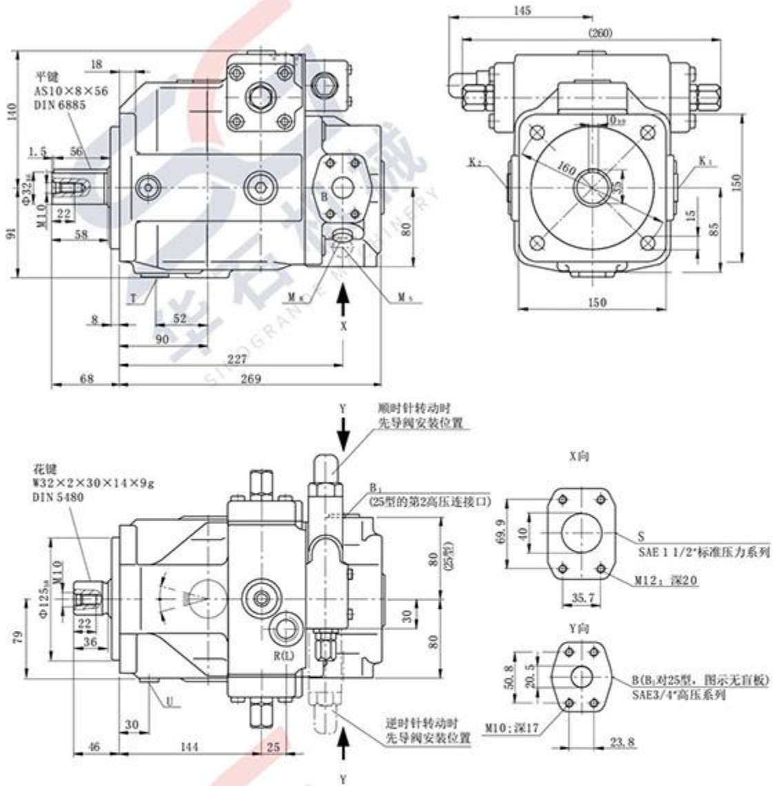
外形尺寸 规格40, 10系列 (图中示例的控制机构是压力控制) Dimension Size 40, Series 10 (Example: pressure control)
