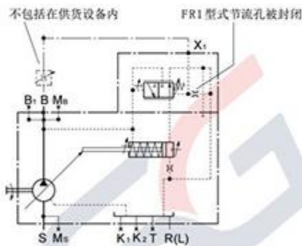
FR 原理图Schematic
